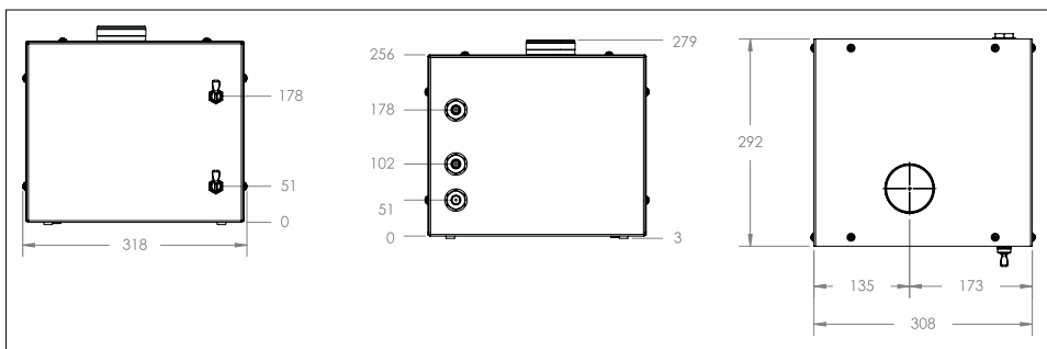
Réservoir 6,5 l - schéma
